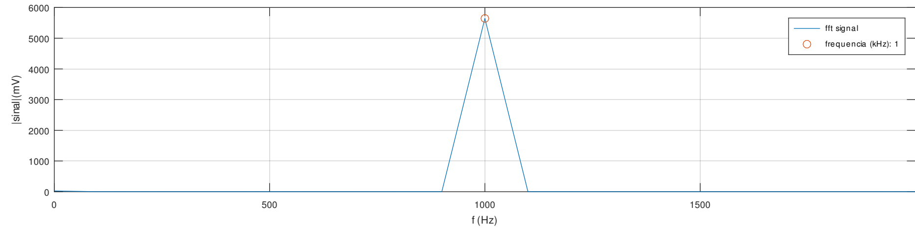
Espectro de amplitudes unilateral X(t) - Saída f=1\text{ kHz} do gerador de sinais com ganho máximo
